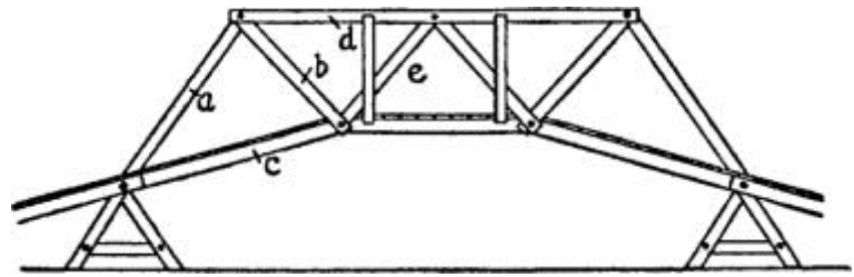
CADRUL PODULUI
